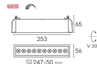
TL-7820.DIR
