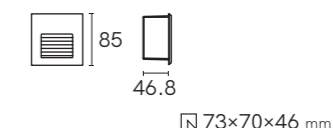
ML-2002.G
