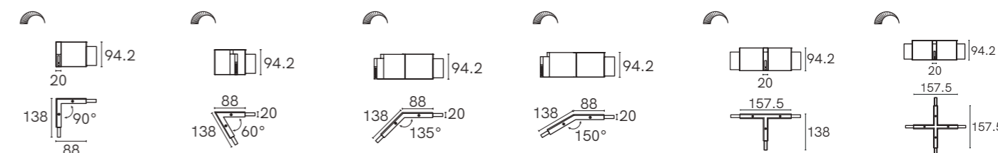
TL-1300.B TL-1300.N
