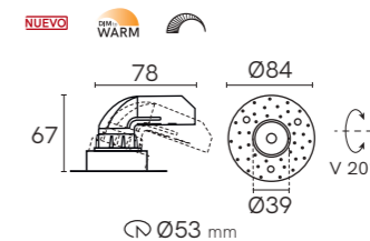
TL-7309.TRDIR
