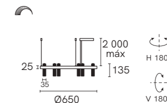
DL-2826
