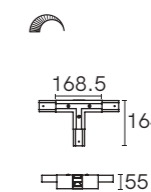
TL-1301.BT TL-1301.NT
