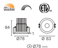
TL-3015
