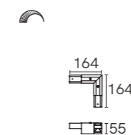
TL-1301 TL-1301.N
