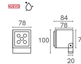
PL-7704.G
