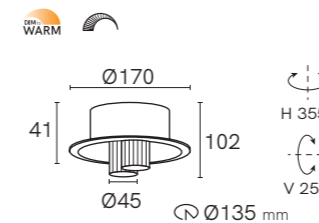
TL-2884
