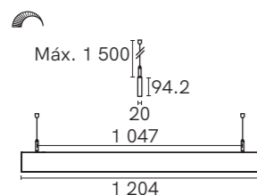
TL-1340.B TL-1340.N
