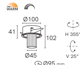
TL-2865
