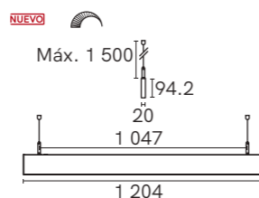
TL-1342.B TL-1342.N
