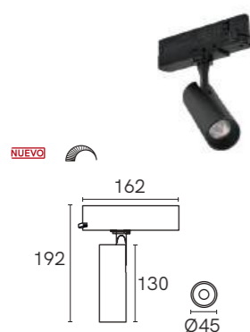
TL-9110.R
