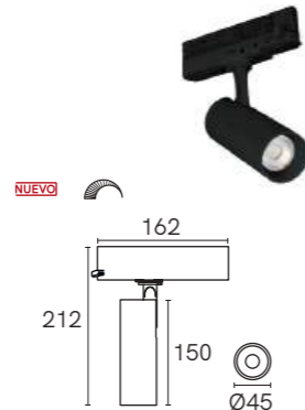
TL-9115.R
