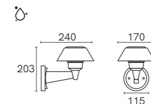
ML-2012.G
