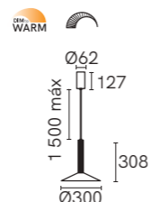
DL-2807
