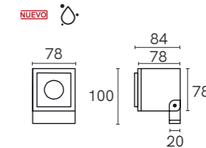
PL-7705.G
