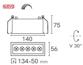
TL-7810.DIR
