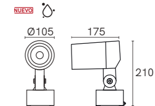
PL-7711.G
